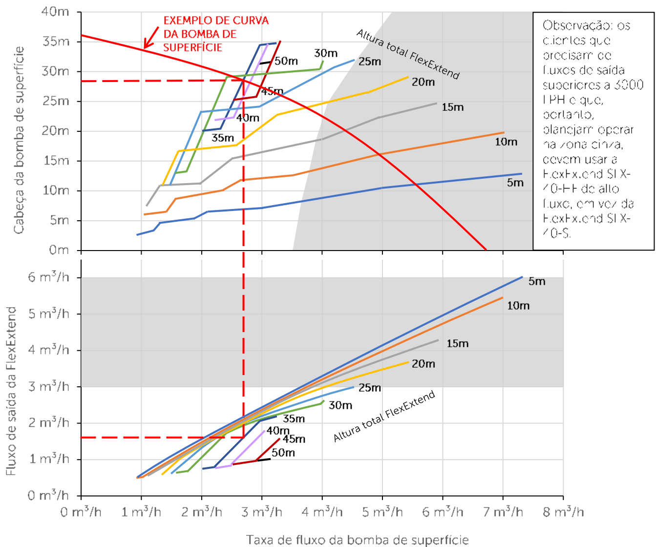
Seleção da bomba de acionamento de superfície para SLX-40-S
